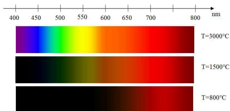
Figure 13.2 – Évolution du spectre continu d'un corps chaud en fonction de la température (Source)
